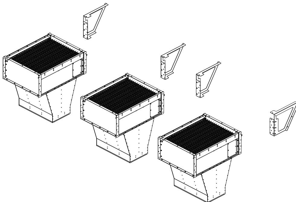
Рисунок 2. Рекомендуемая схема монтажа кронштейнов к группе завес
