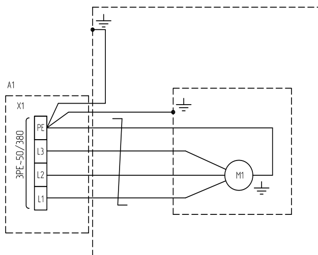
Рисунок 3. Электрическая схема завесы КЭВ-140П8021W
